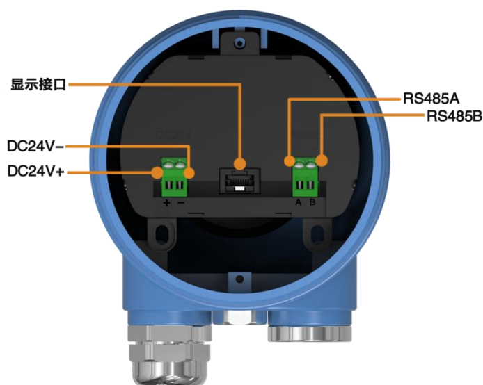
两线制产品接线方式
